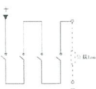
D型接线方式 D connected type
