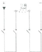
C型接线方式 C connected type
