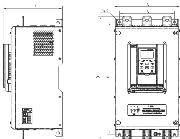
图2.3 Ex9QR3-180-380 ~ Ex9QR3-370-380
