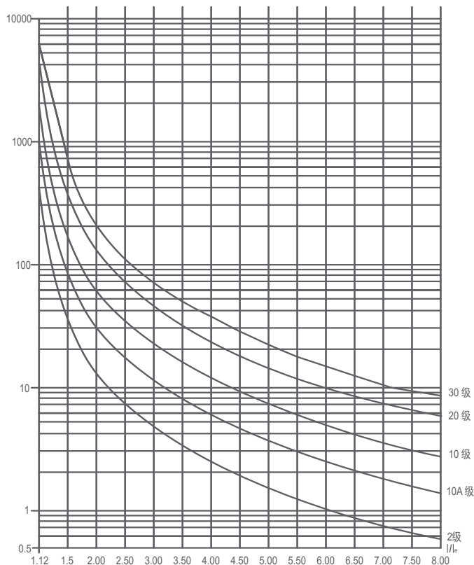
图5.1 标准热过载保护曲线
