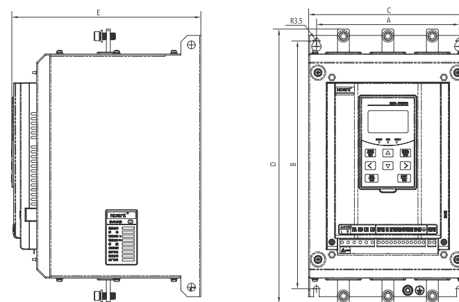
图2.2 Ex9QR3-110-380 ~ Ex9QR3-150-380
