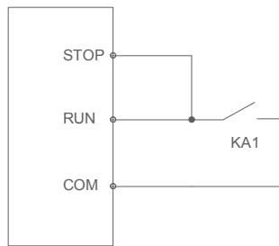
图2.8 两线接法
