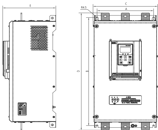
图2.4 Ex9QR3-400-380 ~ Ex9QR3-630-380
