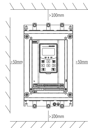
图2.5 安装示意图
