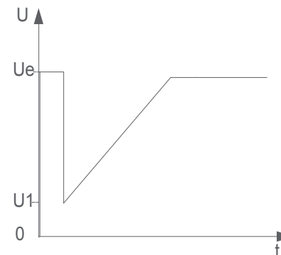
图4.1 突跳时软起动器输出电压示意图
