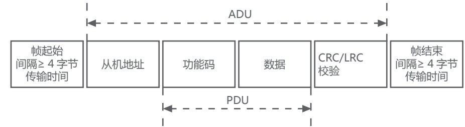
图6.2 协议格式图
